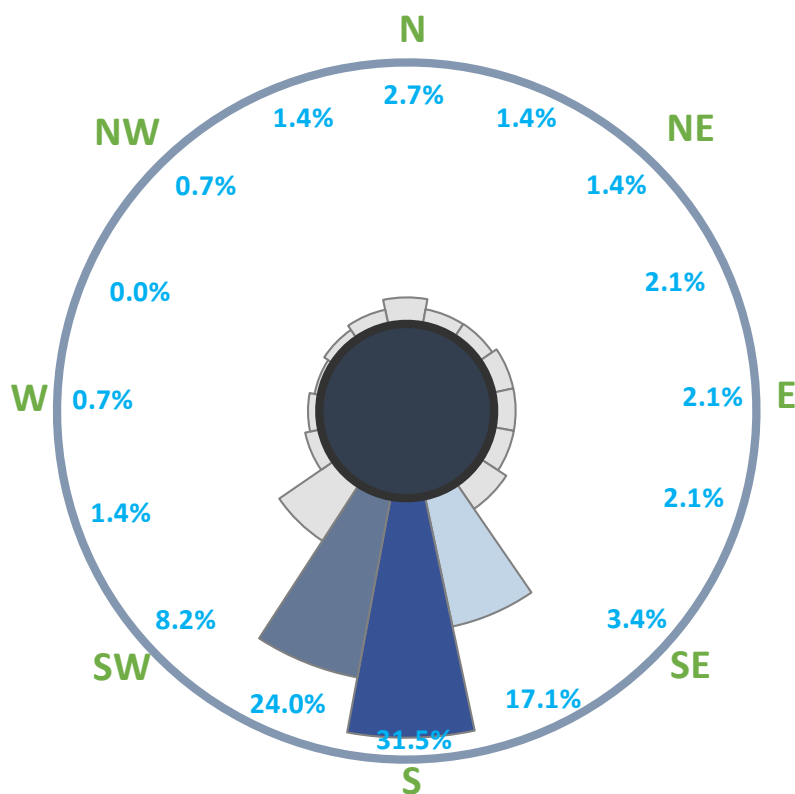
圖 2.2-7 本季水平雷達調查鳥類飛行方向分佈
