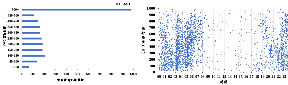
圖 5、113 年冬季（12 月）垂直雷達調查鳥類飛行高度與時間分佈
