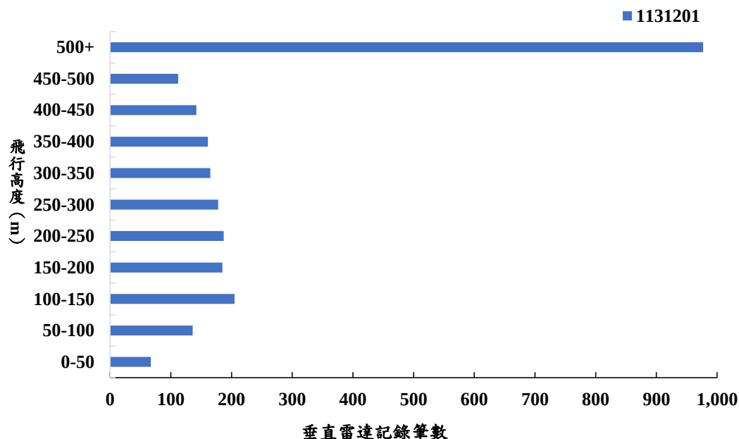
圖 2.2-4 本季垂直雷達調查鳥類飛行高度分佈
