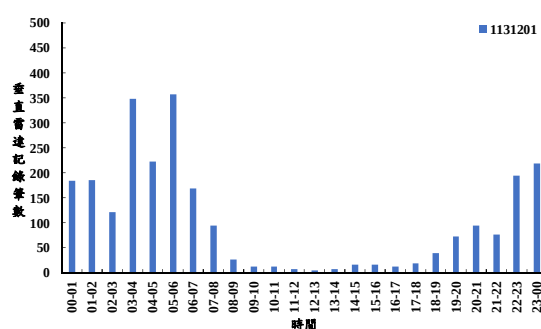
圖 4、113 年冬季（12 月）垂直雷達調查鳥類活動時間分佈
