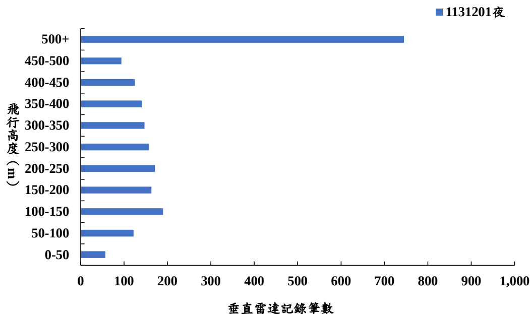
圖 2.2-6 本季垂直雷達調查鳥類飛行高度分佈（夜間）
