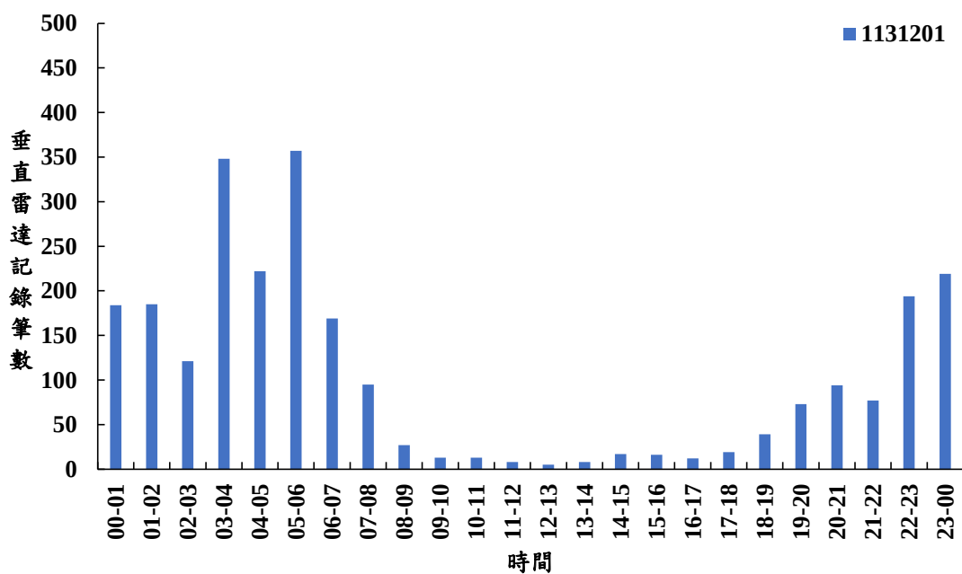
圖 2.2-2 本季垂直雷達調查鳥類活動時間分佈
