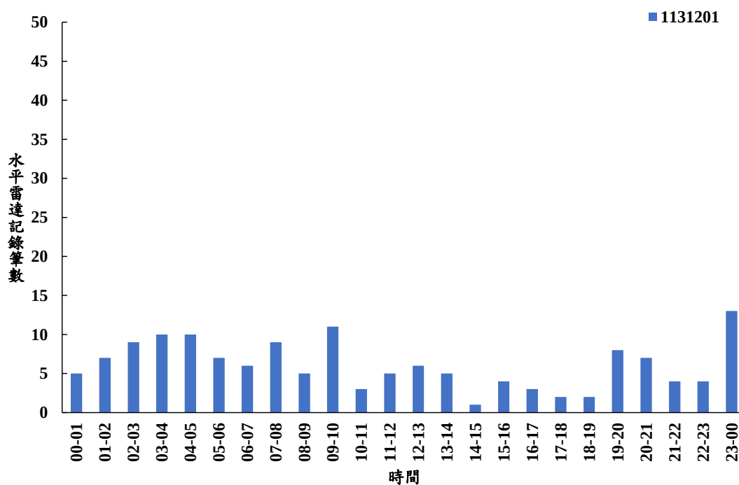
圖 2.2-3 本季水平雷達調查鳥類活動時間分佈
