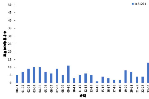
圖 7、113 年冬季（12 月）水平雷達調查時間分佈
