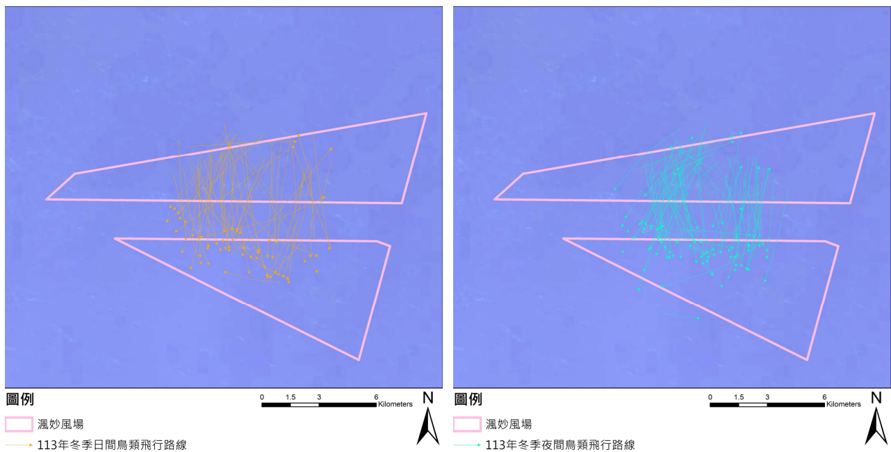
圖 10、113 年冬季（12 月）水平雷達調查日間（左）夜間（右）鳥類飛行軌跡圖
