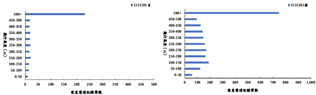
圖 6、113 年冬季（12 月）垂直雷達日間（左）夜間（右）調查鳥類飛行高度分佈
