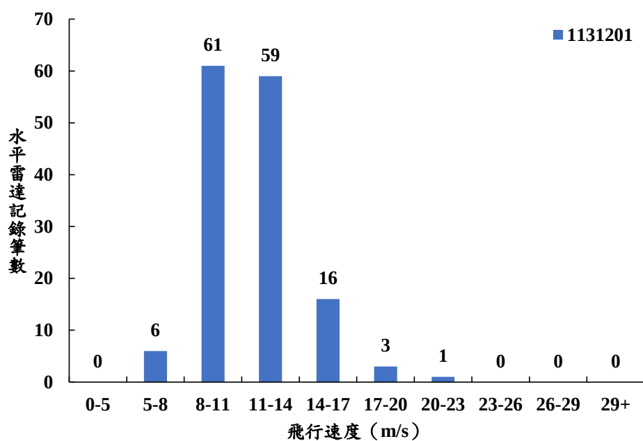
圖 2.2-10 本季水平雷達調查追蹤軌跡之飛行速度
