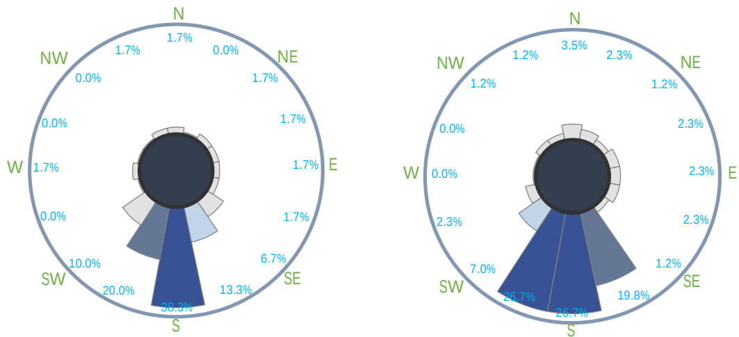
圖 9、113 年冬季（12 月）水平雷達日間（左）及夜間（右）調查鳥類飛行方向
