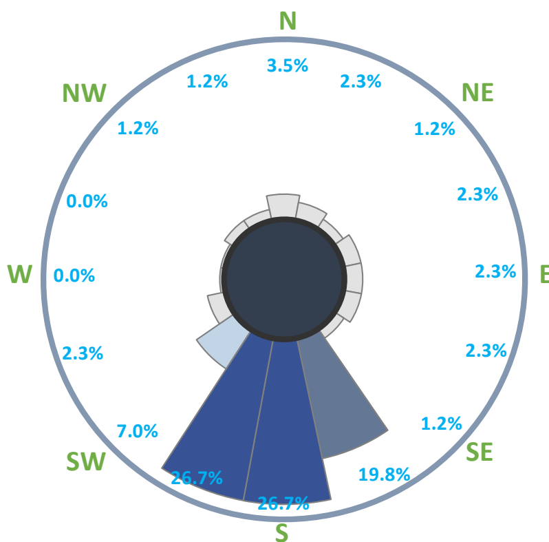
圖 2.2-9 本季水平雷達調查鳥類飛行方向分佈（夜間）
