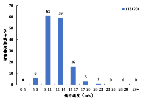
圖 11、113 年冬季（12 月）水平雷達調查追蹤軌跡之飛行速度
