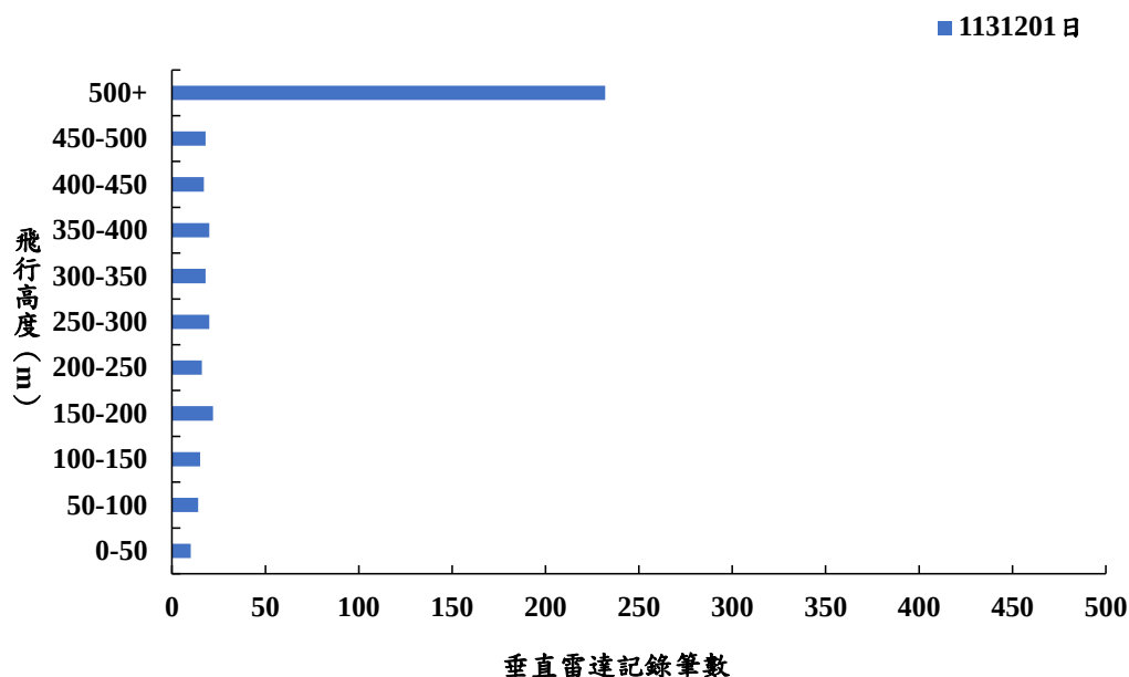
圖 2.2-5 本季垂直雷達調查鳥類飛行高度分佈（日間）
