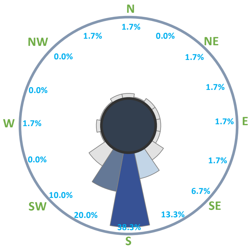
圖 2.2-8 本季水平雷達調查鳥類飛行方向分佈（日間）
