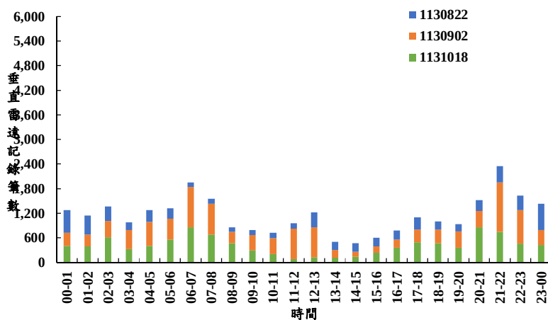
圖 4、113 年秋季 (8 月至 10 月) 垂直雷達調查鳥類活動時間分佈
