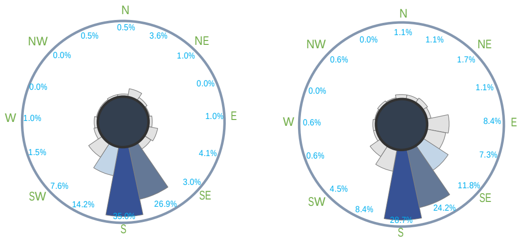
圖 9、113 年秋季（8 月至 10 月）水平雷達日間（左）及夜間（右）調查鳥類飛行方向
