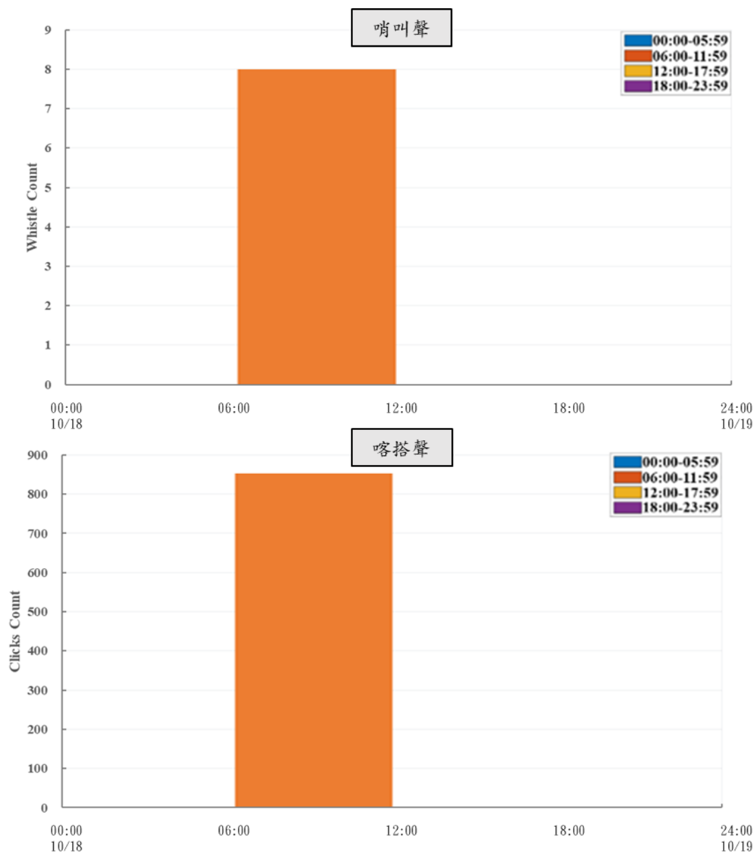
圖 2.1-3 本季 U3 測站鯨豚哨叫聲及喀搭聲訊號辨識結果統計圖
