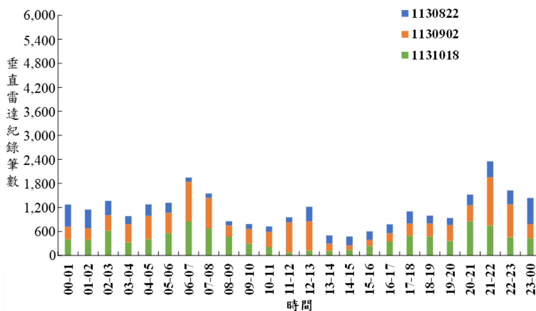
圖 2.2-3 本季垂直雷達調查鳥類活動時間分佈
