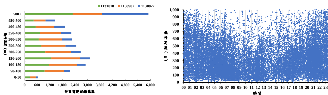
圖 5、113 年秋季 (8 月至 10 月) 垂直雷達調查鳥類飛行高度與時間分佈
