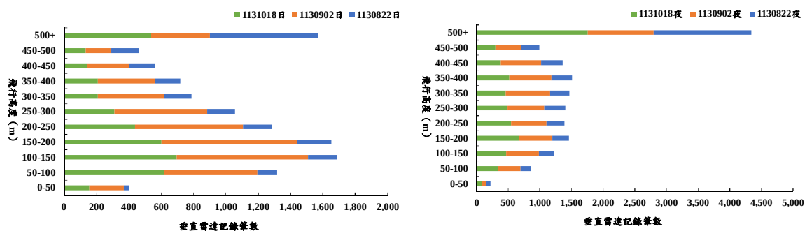
圖 6、113 年秋季 (8 月至 10 月) 垂直雷達日間 (左) 夜間 (右) 調查鳥類飛行高度分佈
