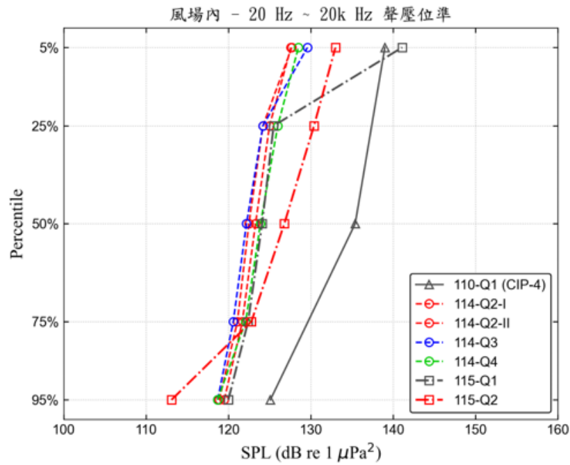
圖 3.1.1-10 歷季 20 Hz~20k Hz 聲壓位準總量
