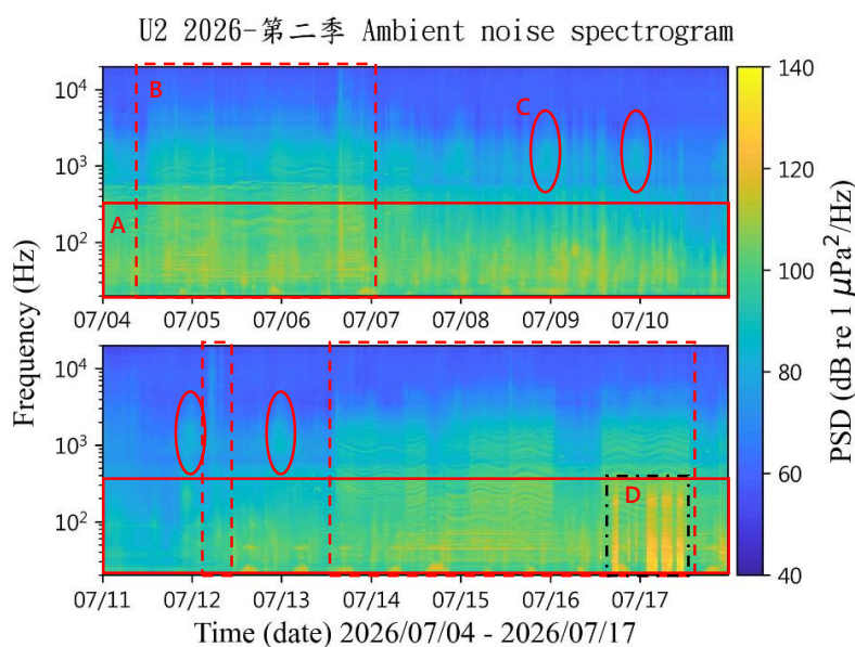
圖 2.10-1 本季環境噪音時頻譜圖
