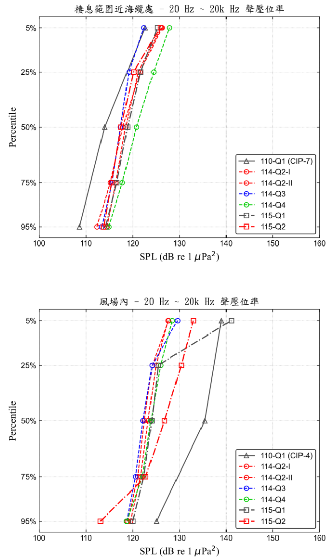
圖 15 各階段 20~20k Hz 聲壓位準總量
