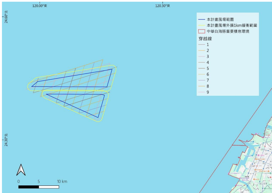
圖 2、本計畫風場鯨豚目視調查穿越線規劃。
