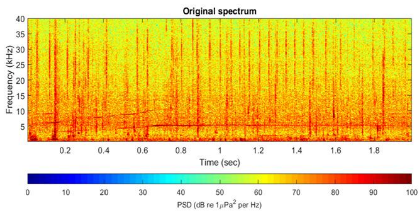
圖 3 利用 STFT 所得之時頻譜圖
