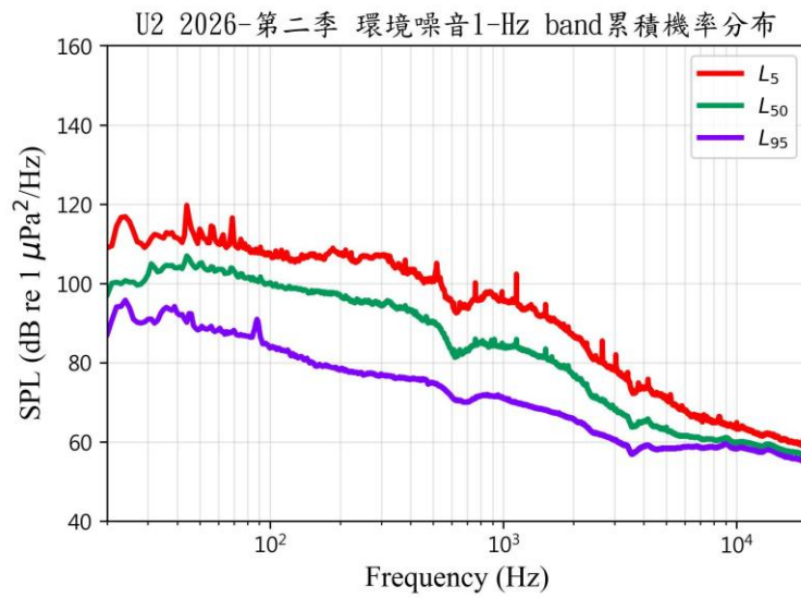
圖 10 U2 1-Hz band 環境噪音頻譜累積機率分佈圖
