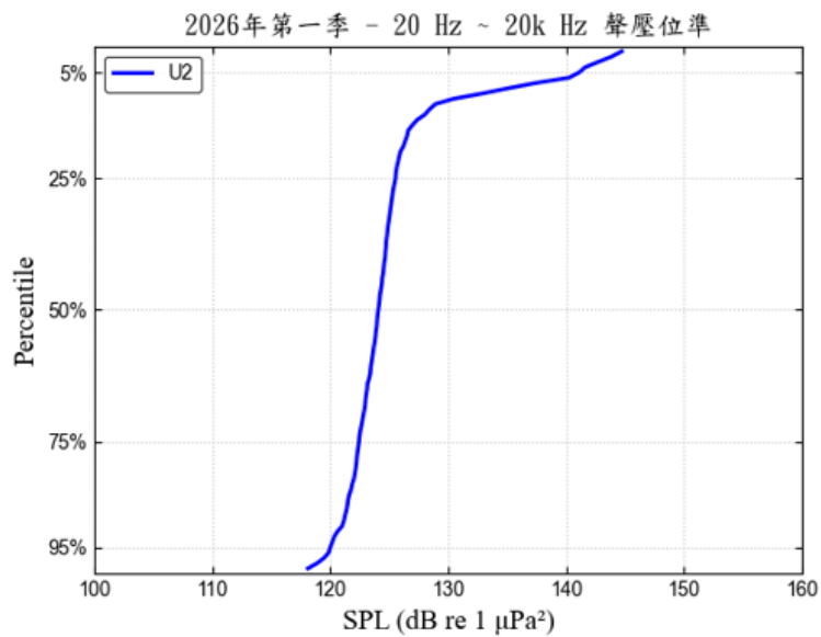
圖 2.10-4 20 Hz~20k Hz 噪音位準總量圖
