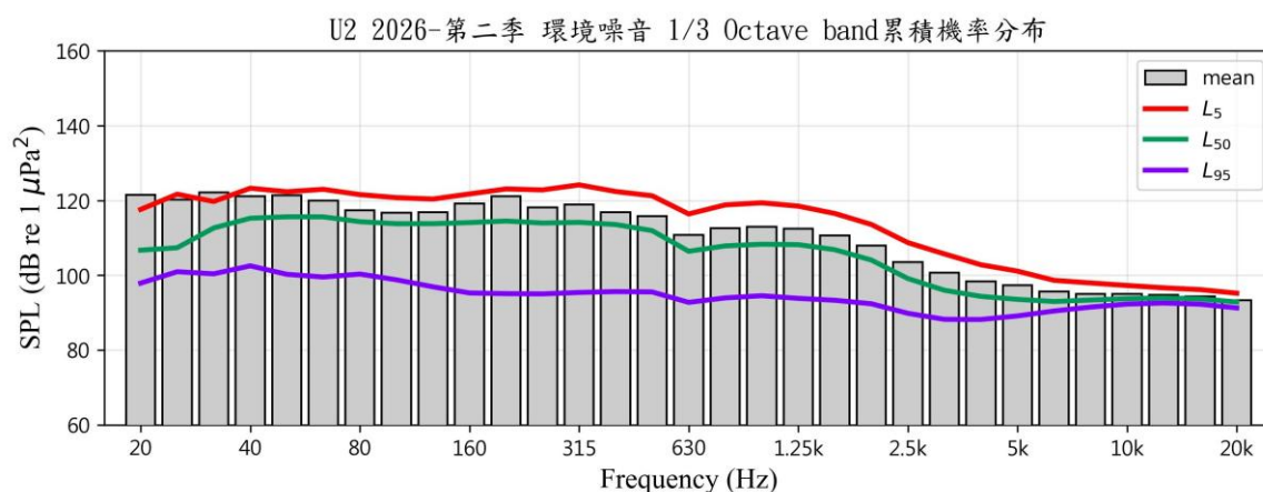
圖 12 U2 環境噪音 1/3 Octave band 頻譜圖
