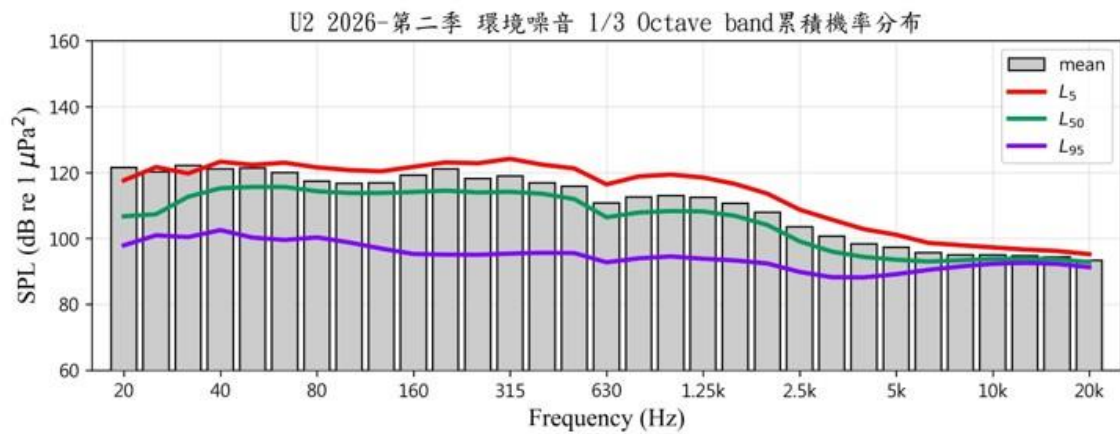
圖 2.10-3 本季 1/3 octave band 水下環境噪音累積機率分布圖
