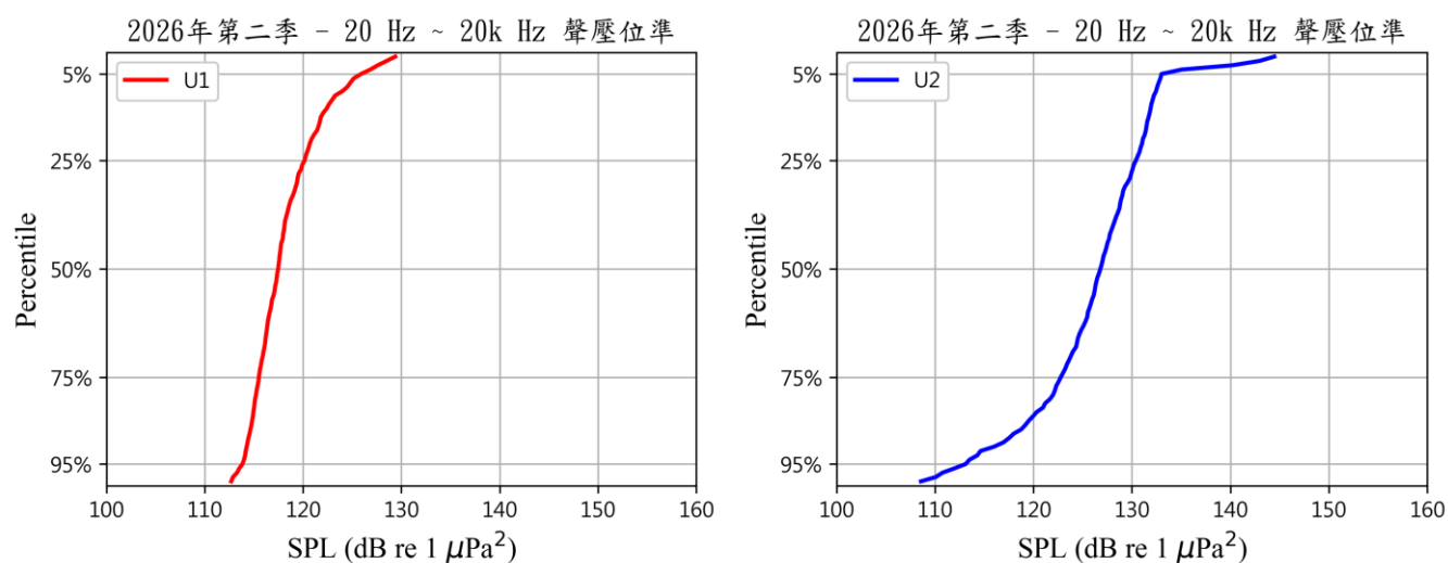
圖 13 20~20k Hz 聲壓位準總量計算
