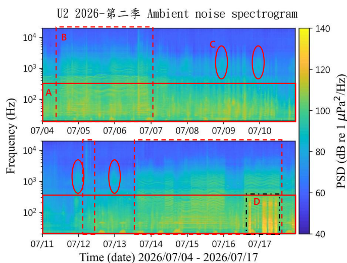
圖 8 U2 環境噪音時頻譜圖
