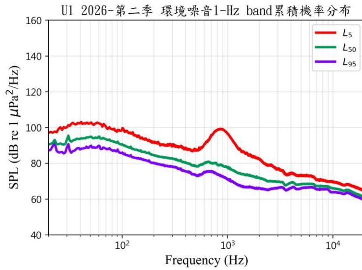
圖 9 U1 1-Hz band 環境噪音頻譜累積機率分佈圖
