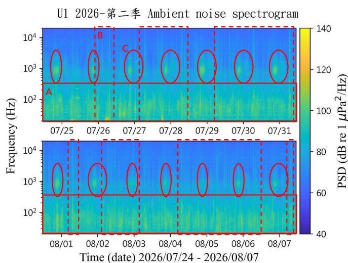
圖 7 U1 環境噪音時頻譜圖
