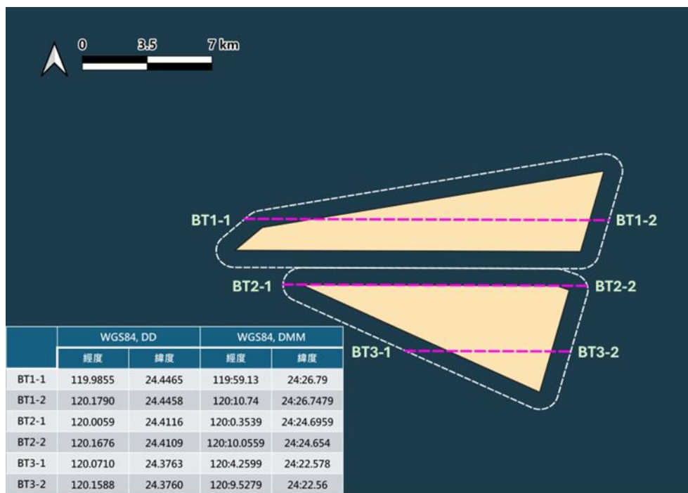
圖 1.3.3-5 本計畫海上鳥類目視穿越線示意圖
