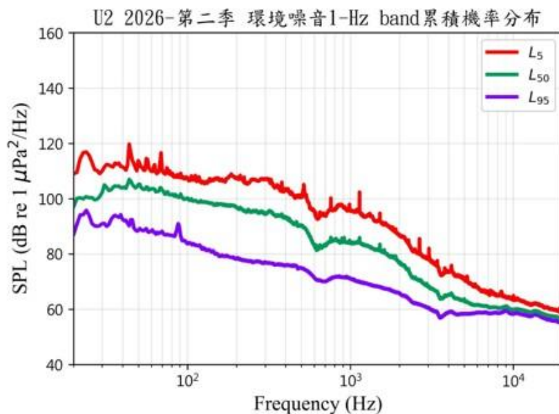
圖 2.10-2 本季 1-Hz band 水下環境噪音累積機率分布圖
