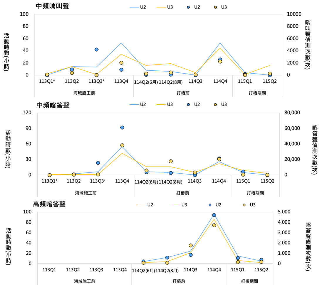
圖 3.1.1-9 歷季水下聲學監測結果趨勢圖
