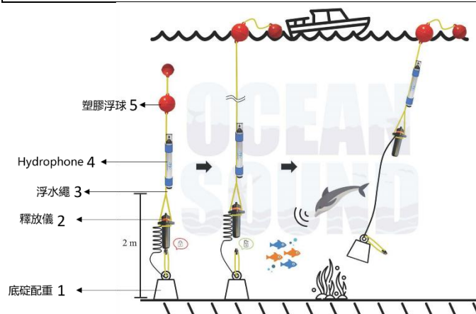
圖 1.3.3-12 釋放儀(Release)系統配置示意圖
