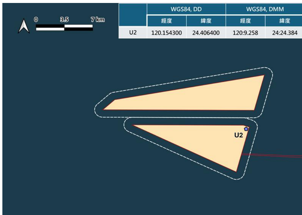
圖 1.3.3-13 本計畫水下噪音監測點位示意圖
