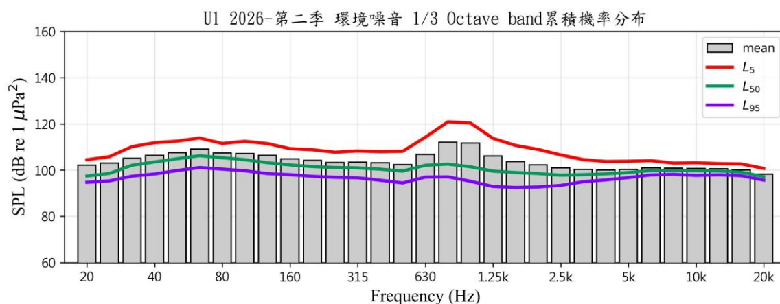
圖 11 U1 環境噪音 1/3 Octave band 頻譜圖
