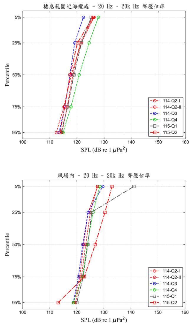
圖 14 各季 20~20k Hz 聲壓位準總量
